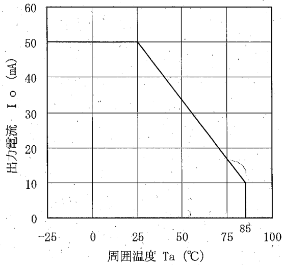
(图1) 出力電流低減曲線
