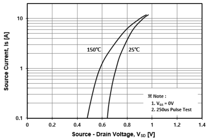
Fig. 4 I_S - V_{SD}
