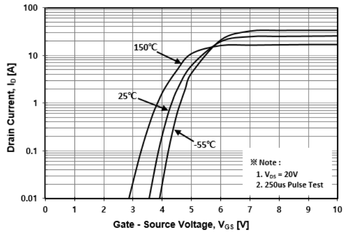
Fig. 2 I_D - V_{GS}
