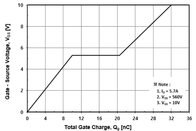
Fig. 6 V_{GS} - Q_g
