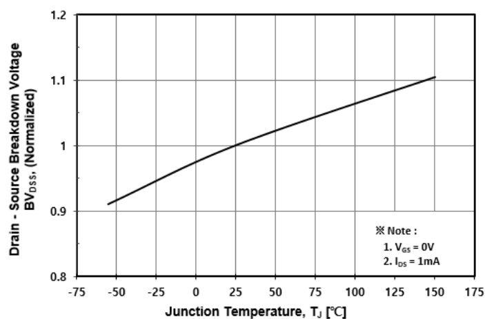
Fig. 7 BV_{DSS} - T_J
