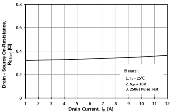
Fig. 3 R_{DS(ON)} - I_D
