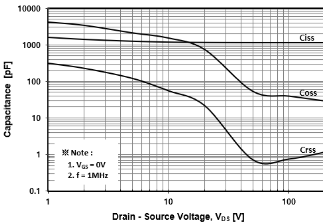
Fig. 5 Capacitance - V_{DS}
