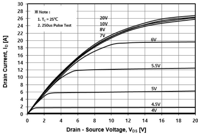
Fig. 1 I_D - V_{DS}
