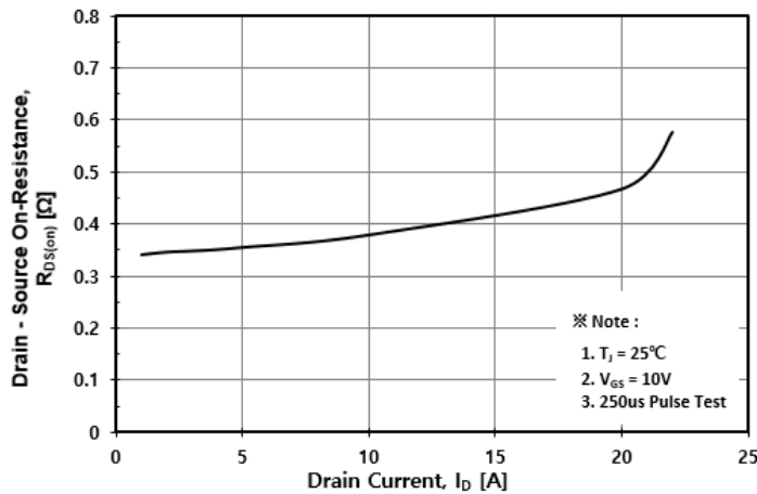
Fig. 3 R_{DS(ON)} - I_D
