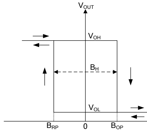
图4. 磁场特性
