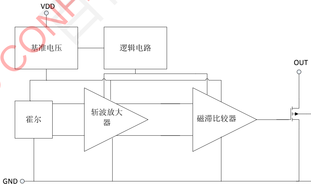
图 3. 功能框图
