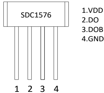
图 2. 管脚排布
