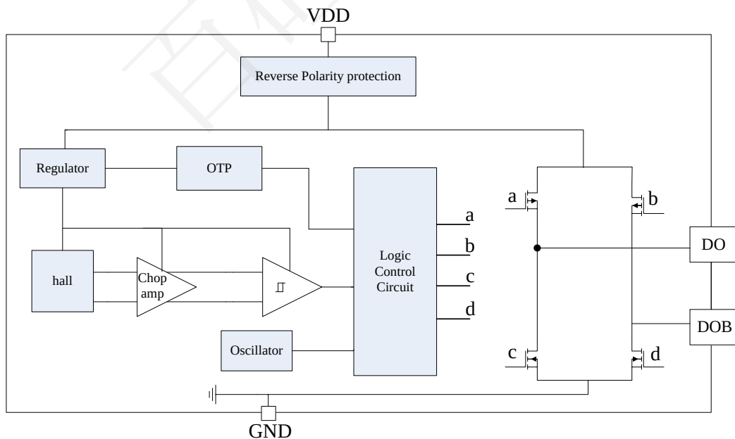
图 3. 功能框图
