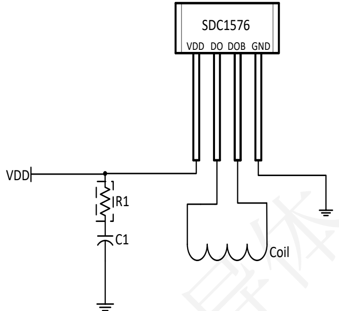
图 6. 典型应用图
