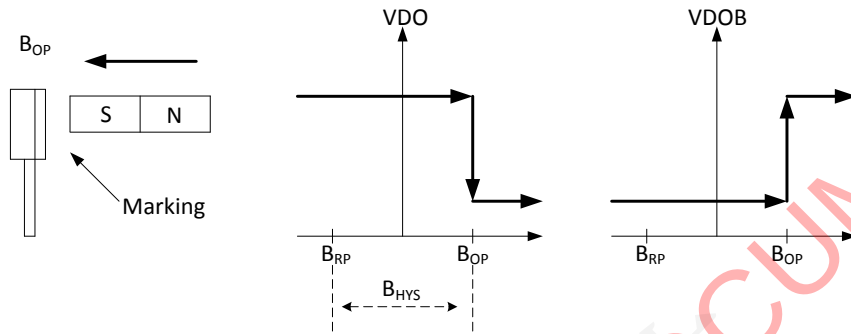
图 5. 磁场特性图
