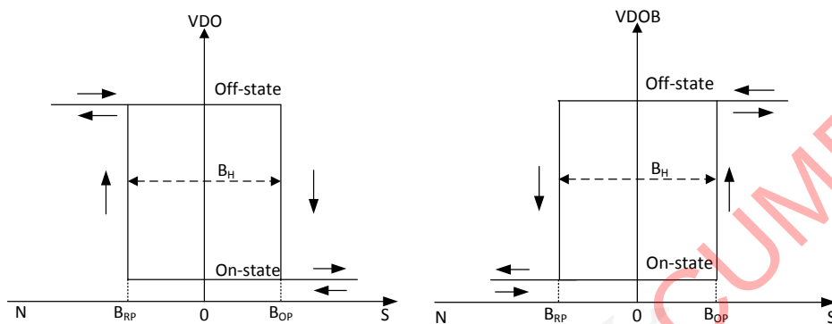
图 4. 磁场特性
