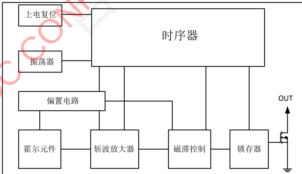
图 3. 功能框图
