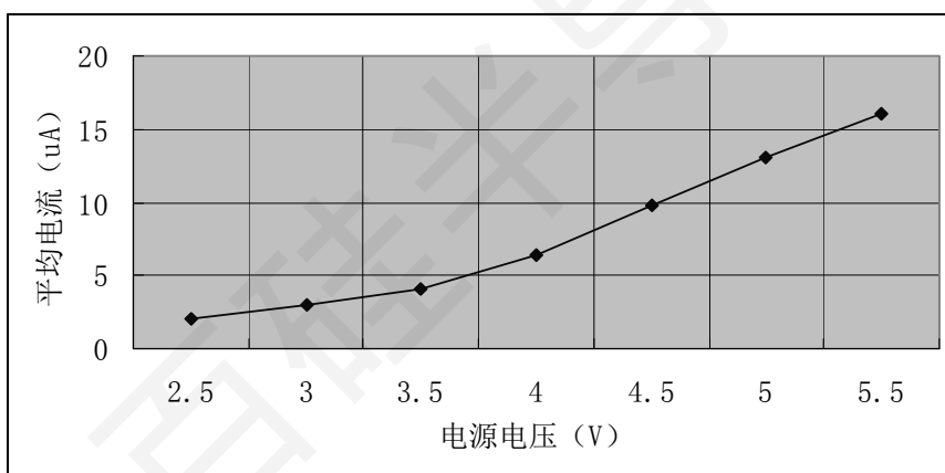
图 4 平均电流相对于电源电压变化曲线 ( Temp=25^{\circ}C )
