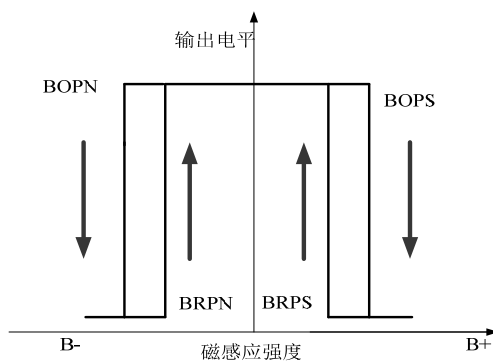
图 5 磁场特性图
