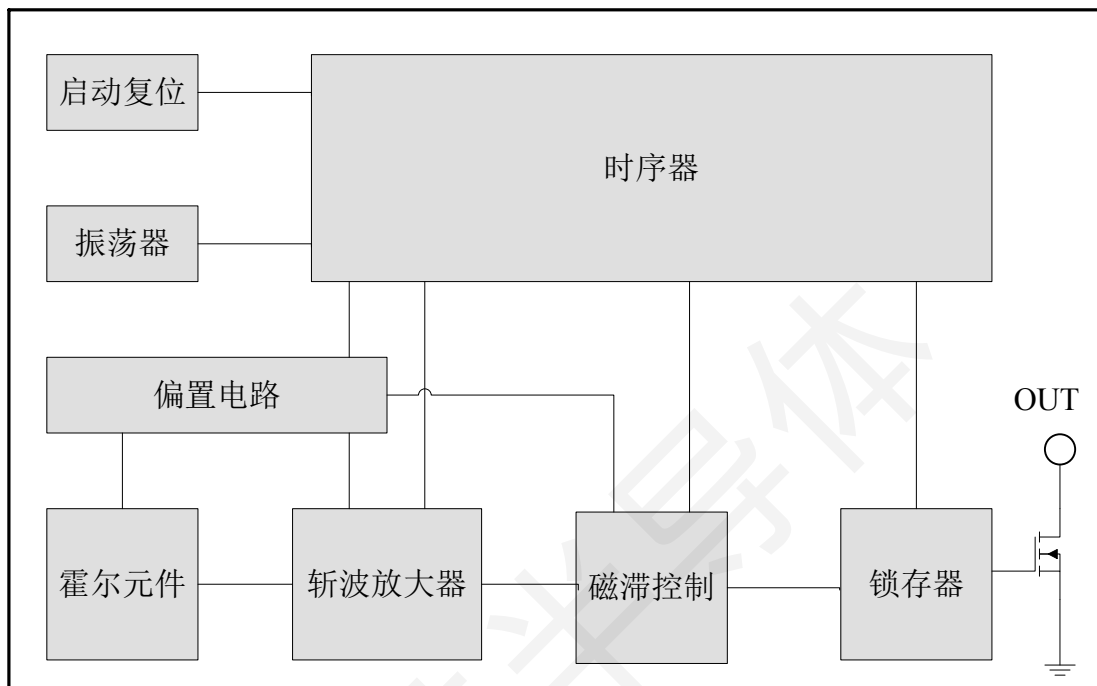
图 2 功能框图
