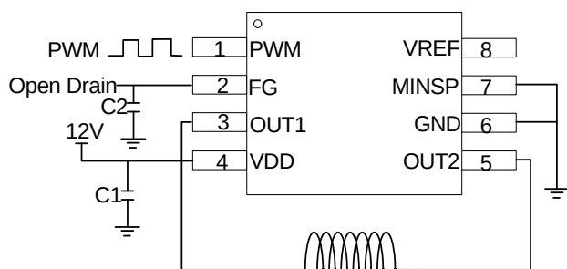
(1)PWM 控制风扇 (无最小速度设置)
