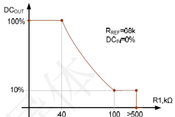
图 6. MINSP 电阻调速
