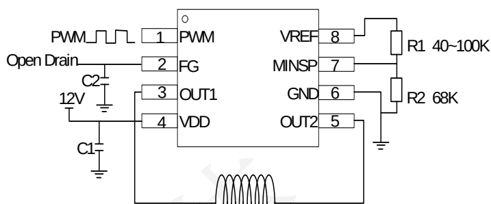
(4)PWM 和 R 双控调速模式
