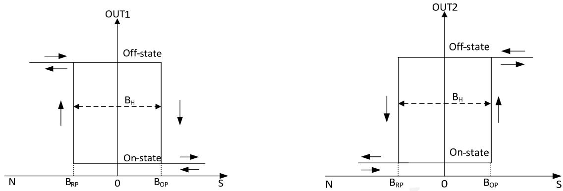
图 4. 输出 VS 磁场特性
