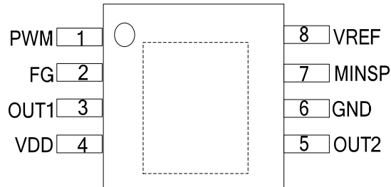
图 2. 管脚排布
