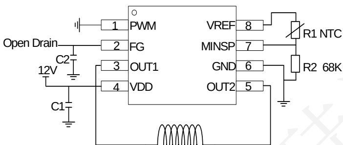
(3)热敏电阻控制风扇
