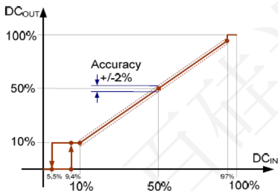
图 5. PWM 调速
