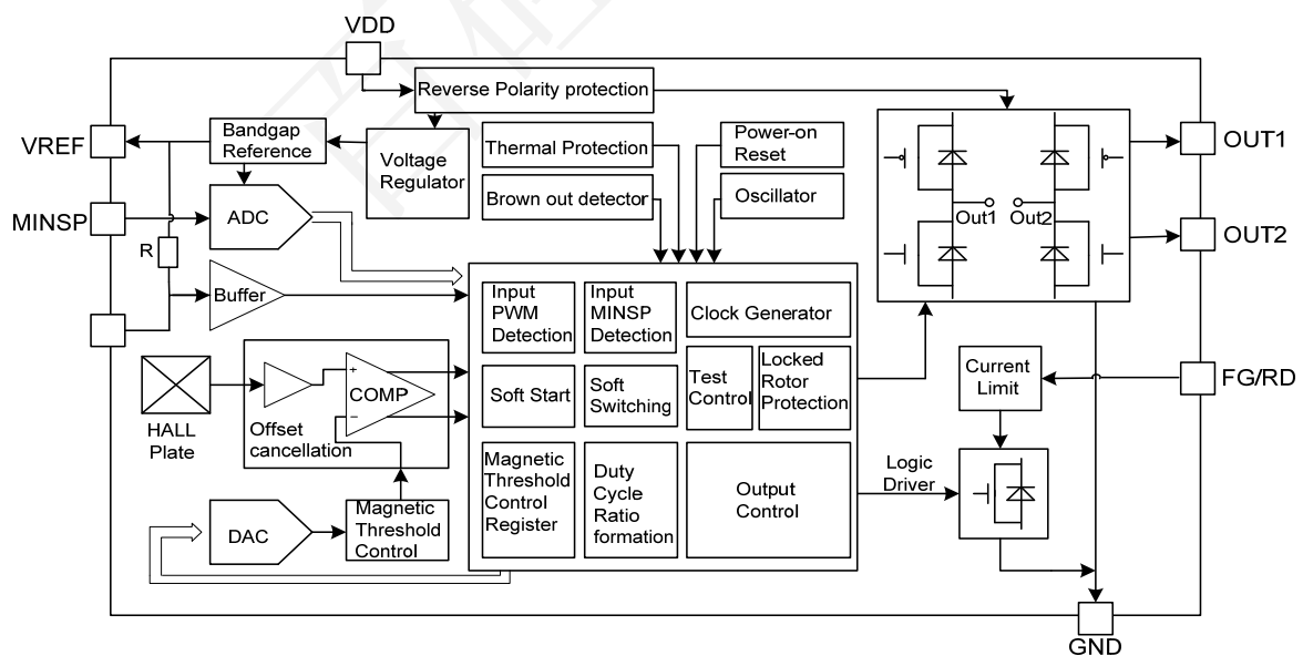
图 3. 功能框图
